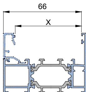
HUECOS DE JUNQUILLO PARA MARCO:
