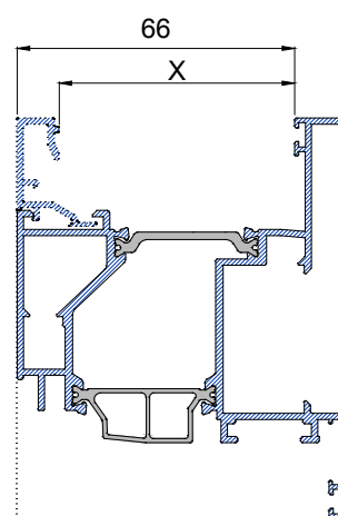
HUECOS DE JUNQUILLO PARA HOJA:
