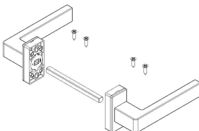
Manilla puerta Kora 02563 Door handle Kora 02563
