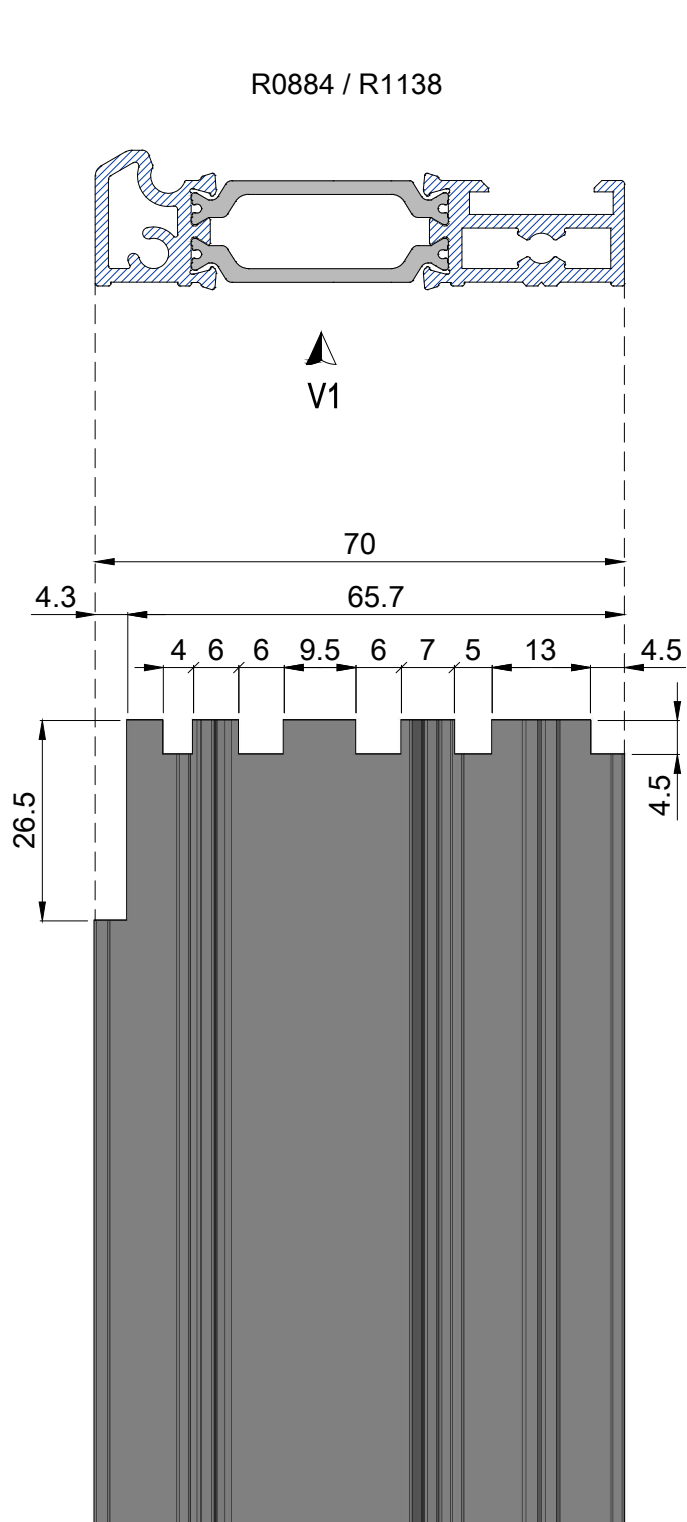
Mecanizado perfil suelo V1 Retestado con fresa A498101* 1:1
