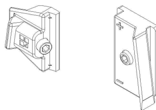
Punto adicional lado bisagras 01350 Fastening element Futura
