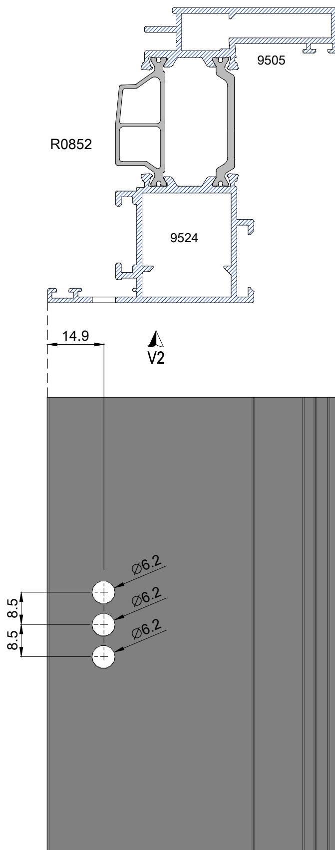
Mecanizado cremona NP M6
