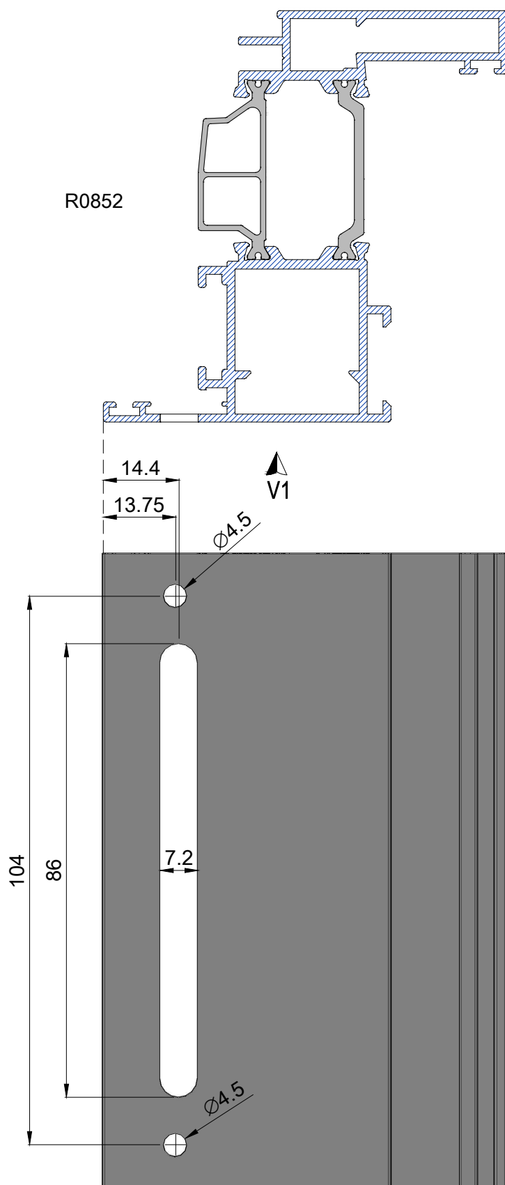
Mecanizado cremona M1
