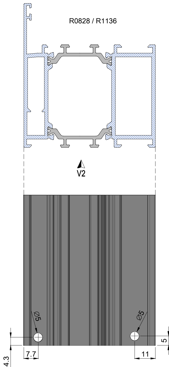
Mecanizado marco V2 1:1
