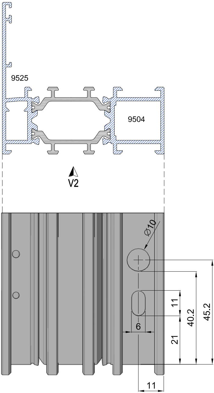
Mecanizado escuadra A495467B M4 V2 1:1
