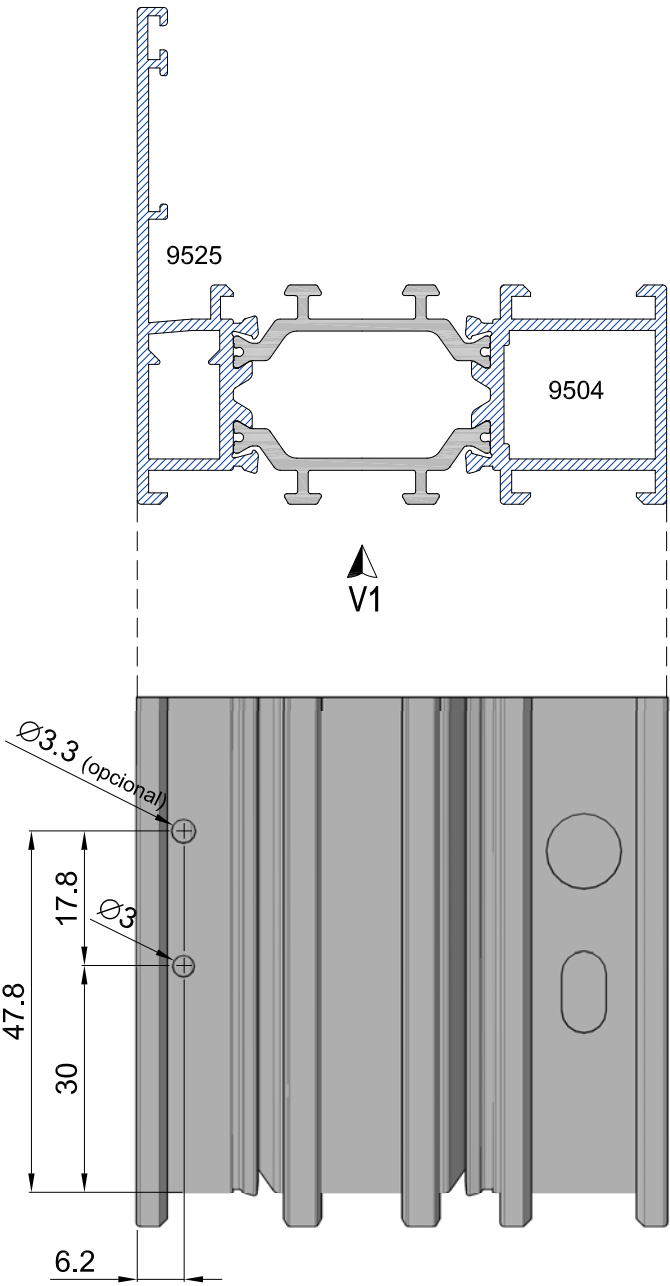
Mecanizado escuadra exterior M3 V1 1:1
