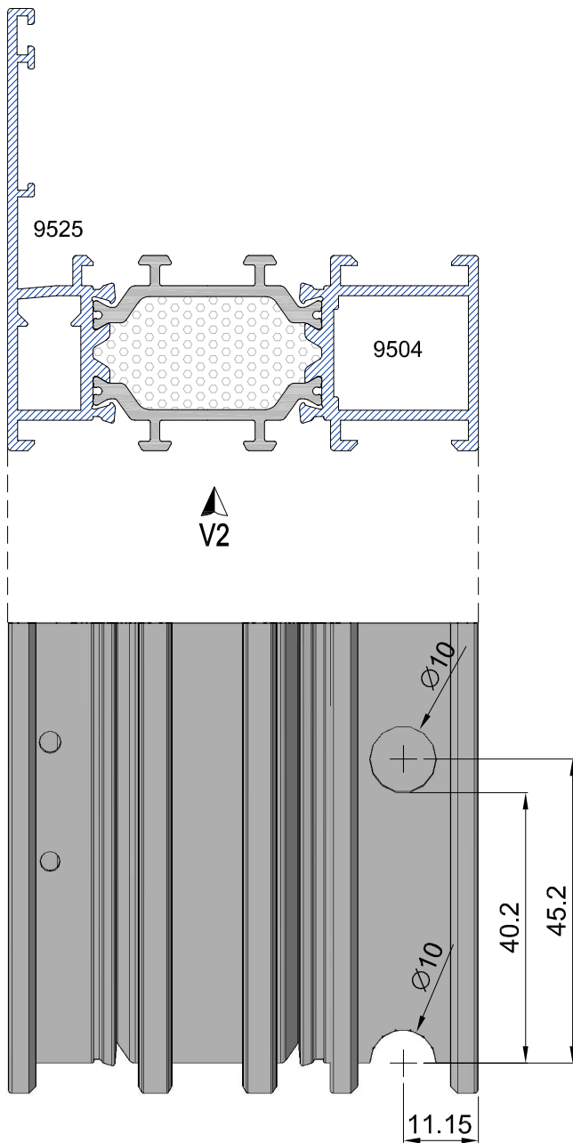
Mecanizado escuadra A495346B Opcional
