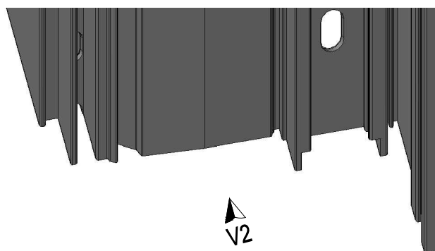
Mecanizado pestañas canal herraje M2
