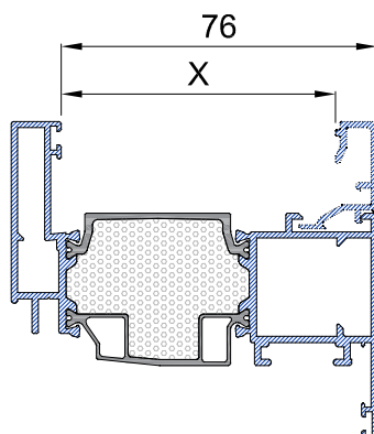
HUECOS DE JUNQUILLO PARA HOJA:
