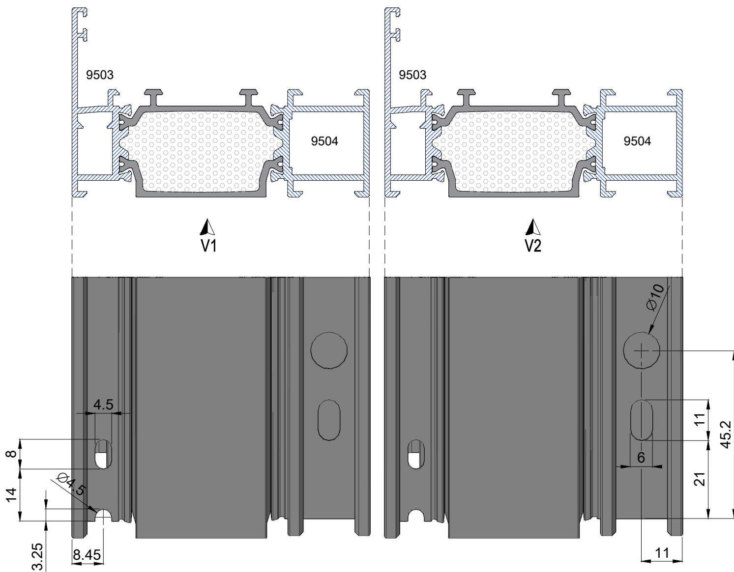
Mecanizado escuadra exterior M3
