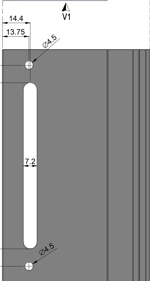
Mecanizado cremona M1
