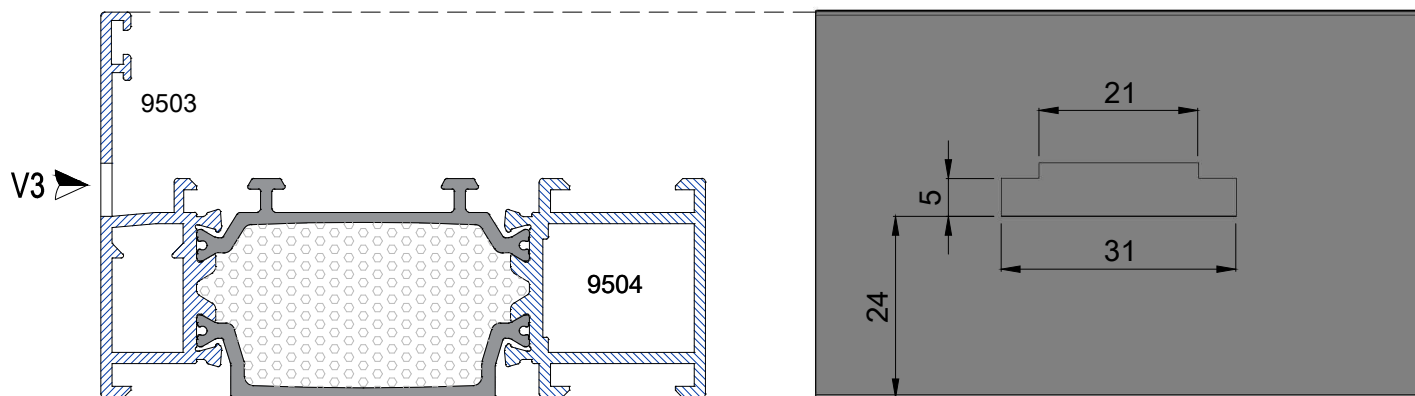
Mecanizado desagüe M7
