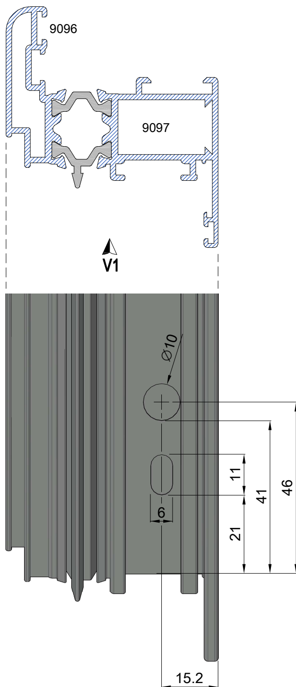
Mecanizado escuadra tetón retráctil M4
