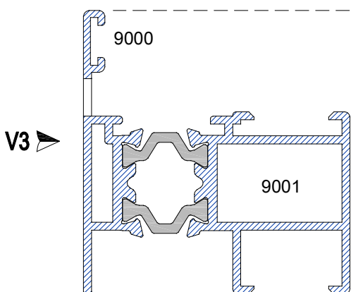
Mecanizado escuadra tetón retráctil M4
