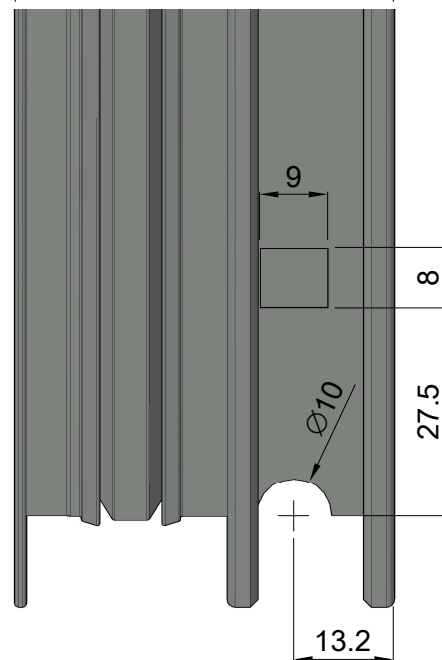
Mecanizado escuadra de vértice M3
