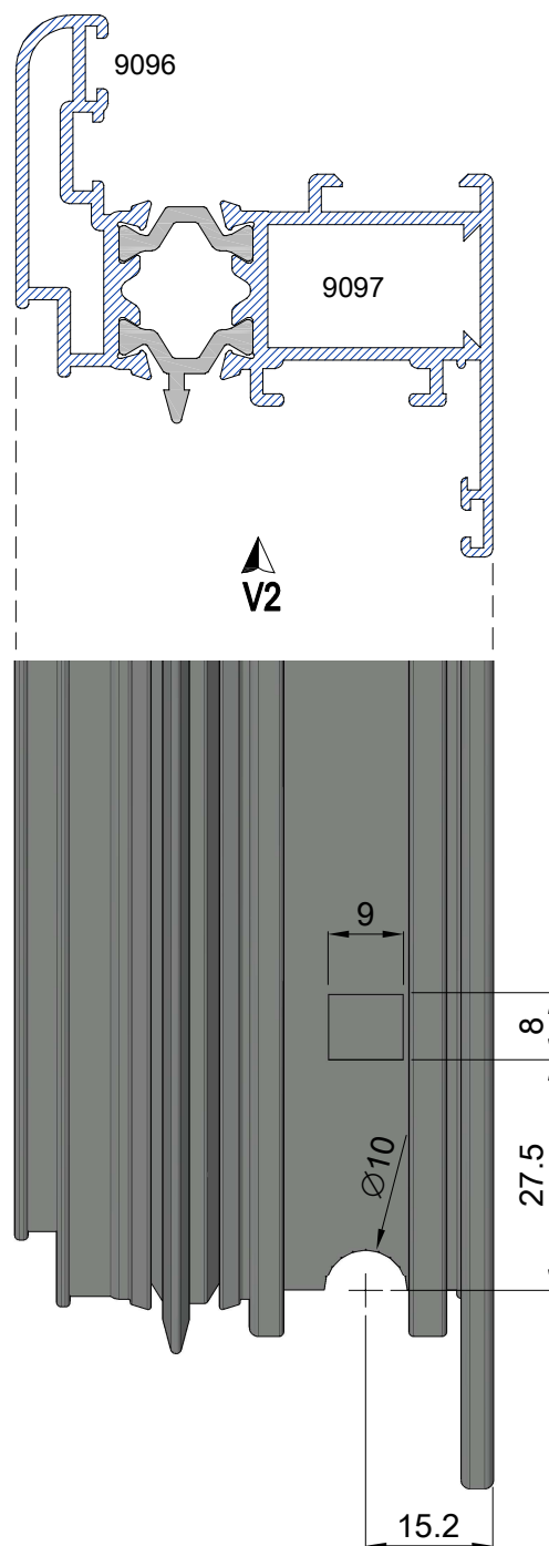
Mecanizado escuadra de vértice M3
