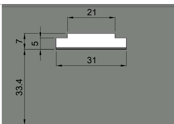
Mecanizado desagüe marco M7
