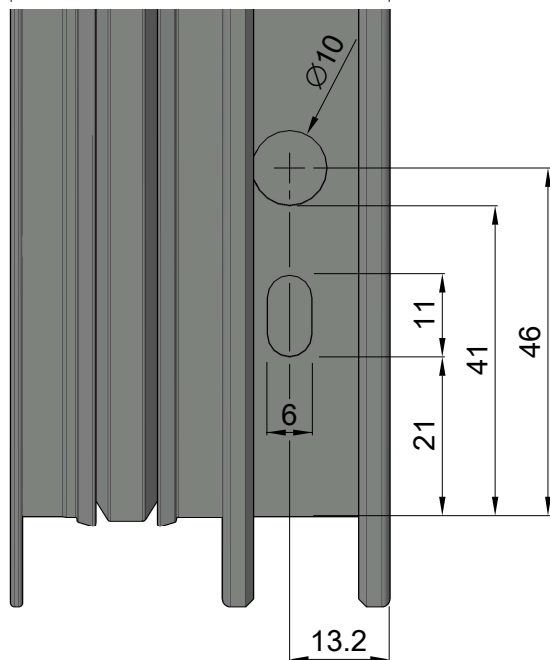
Mecanizado escuadra tetón retráctil M4
