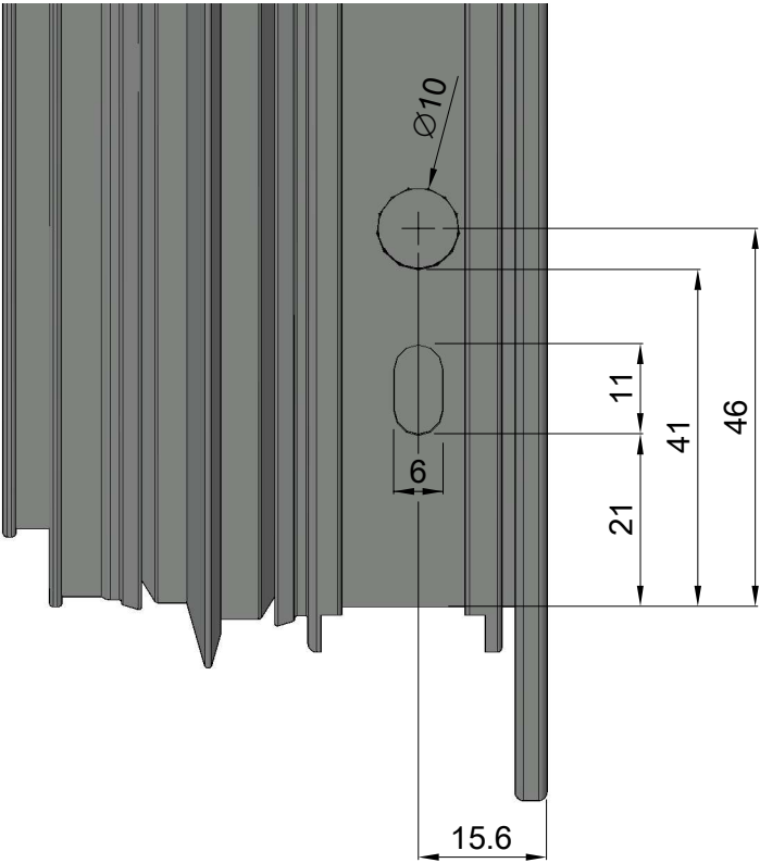
Mecanizado escuadra tetón retráctil M4
