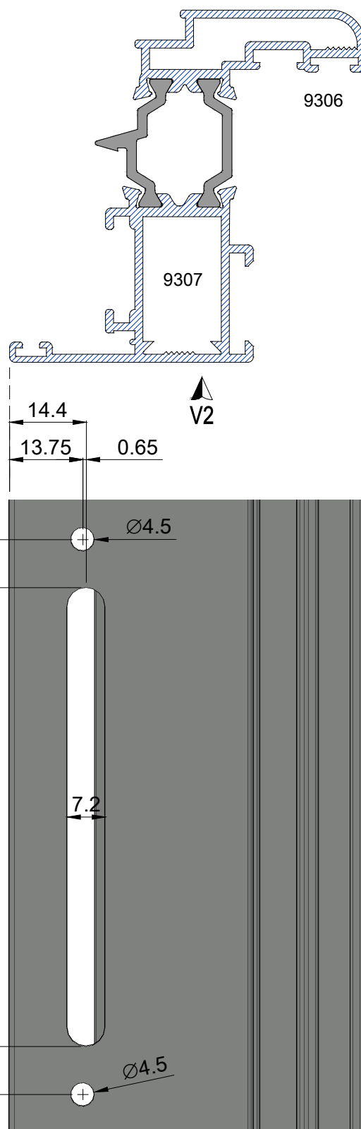
Mecanizado cremón M1
