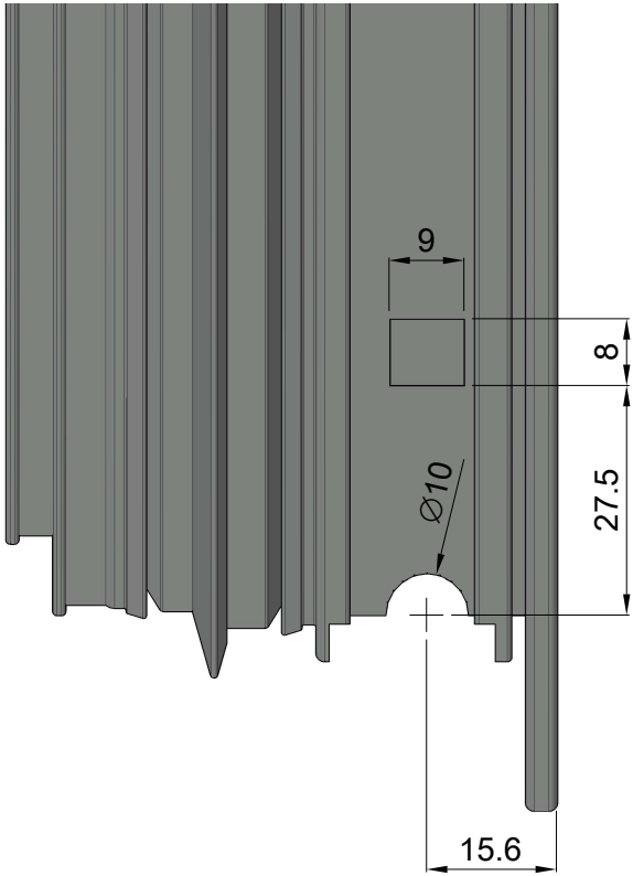
Mecanizado escuadra de vértice M3
