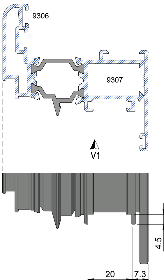
Mecanizado pestañas canal herraje M2
